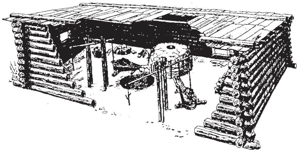
Рис. 1. Реконструкция древнеудмуртской кузницы (по материалам городища Иднакар)
